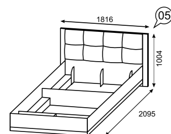
Каркас кровати 1600 (под ПМ и ортопед. основание)
