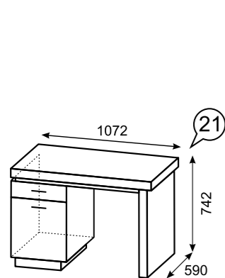
21 Стол письменный (правое и левое исполнение)
