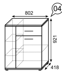
Тумба комбинированная
