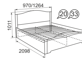
Кровать одинарная (900) / (1200) (с латами и б/матр.)
