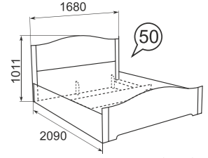
Каркас кровати (1600) (под ПМ и ортопед. основание)
