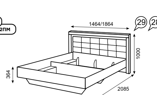
28 Каркас кровати (1200/1600) (под ПМ и ортопед. основание) (с мягким элементом)
